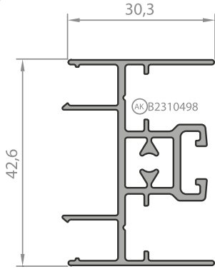
Kenet Profili - Hook
