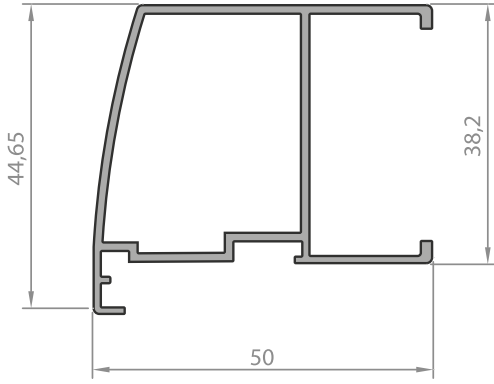
Orta Kilitleme Profili - Center Locking Profili
