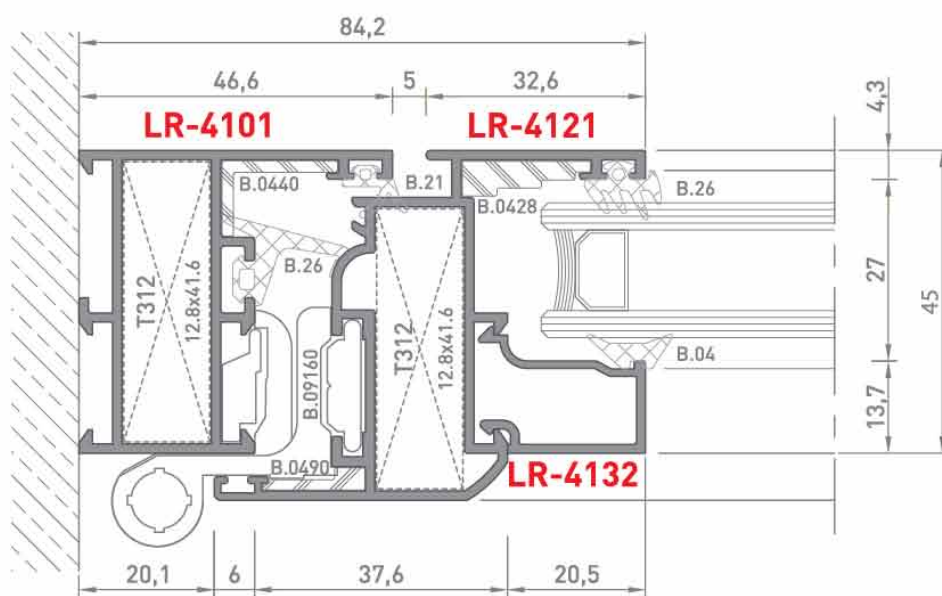
3.3 Detayı Details
