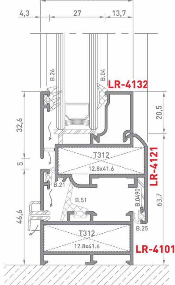
2.2 Detayı Details
