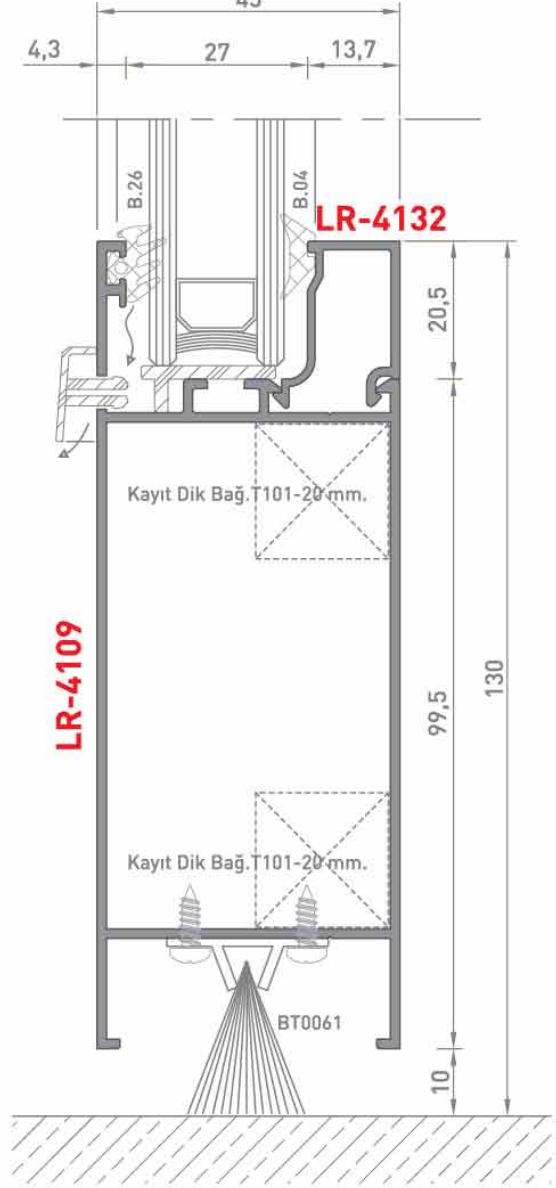
7.7 Detayı Details
