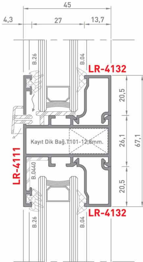
6.6 Detayı Details
